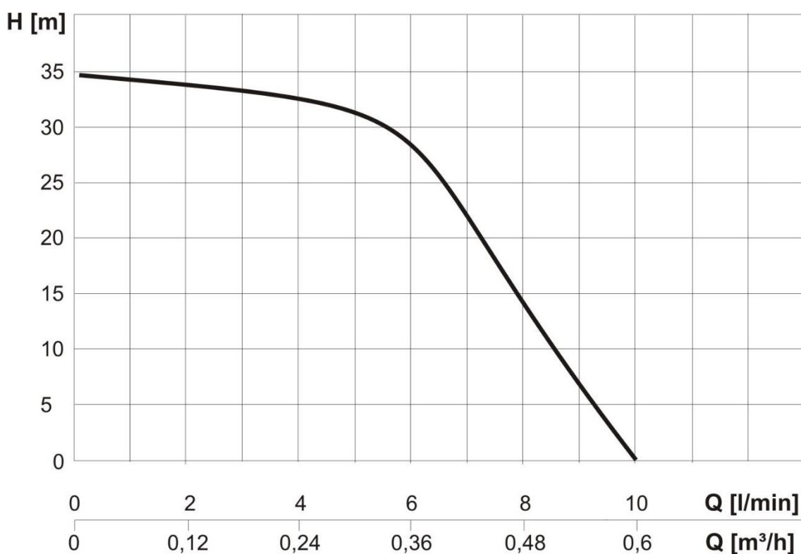
Charakterystyka pracy pompy AquaMatic Domestic Eco 10
